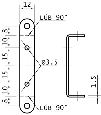
Bracfráma
