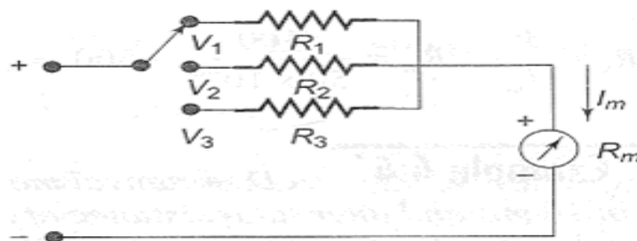
fig. 4. a. (iii) Multirange Voltmeter
